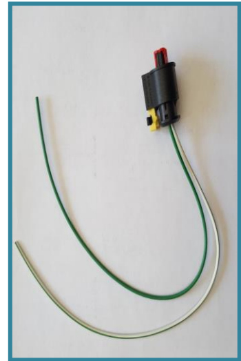
CONECTOR DE INYECTOR CLAVE: 06LB50010109
