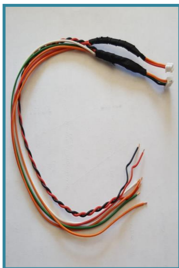
CONECTOR DE COMUTADOR CLAVE: DE512252
